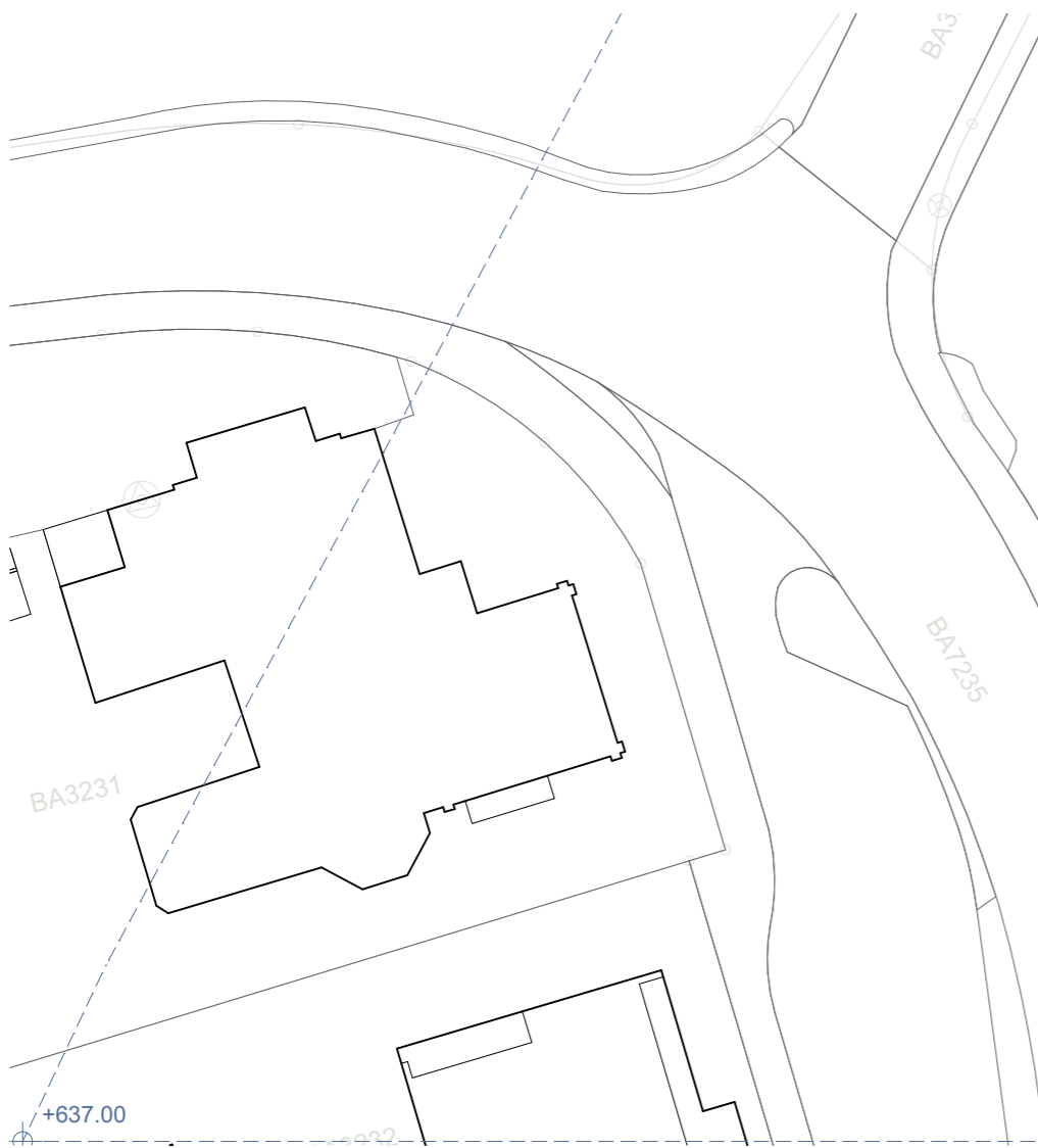
Isohypsen des mutmasslichen mittleren Grundwasserspiegels gem. Messungen der Firma Jäckli Geologie AG (17.11.2021)
