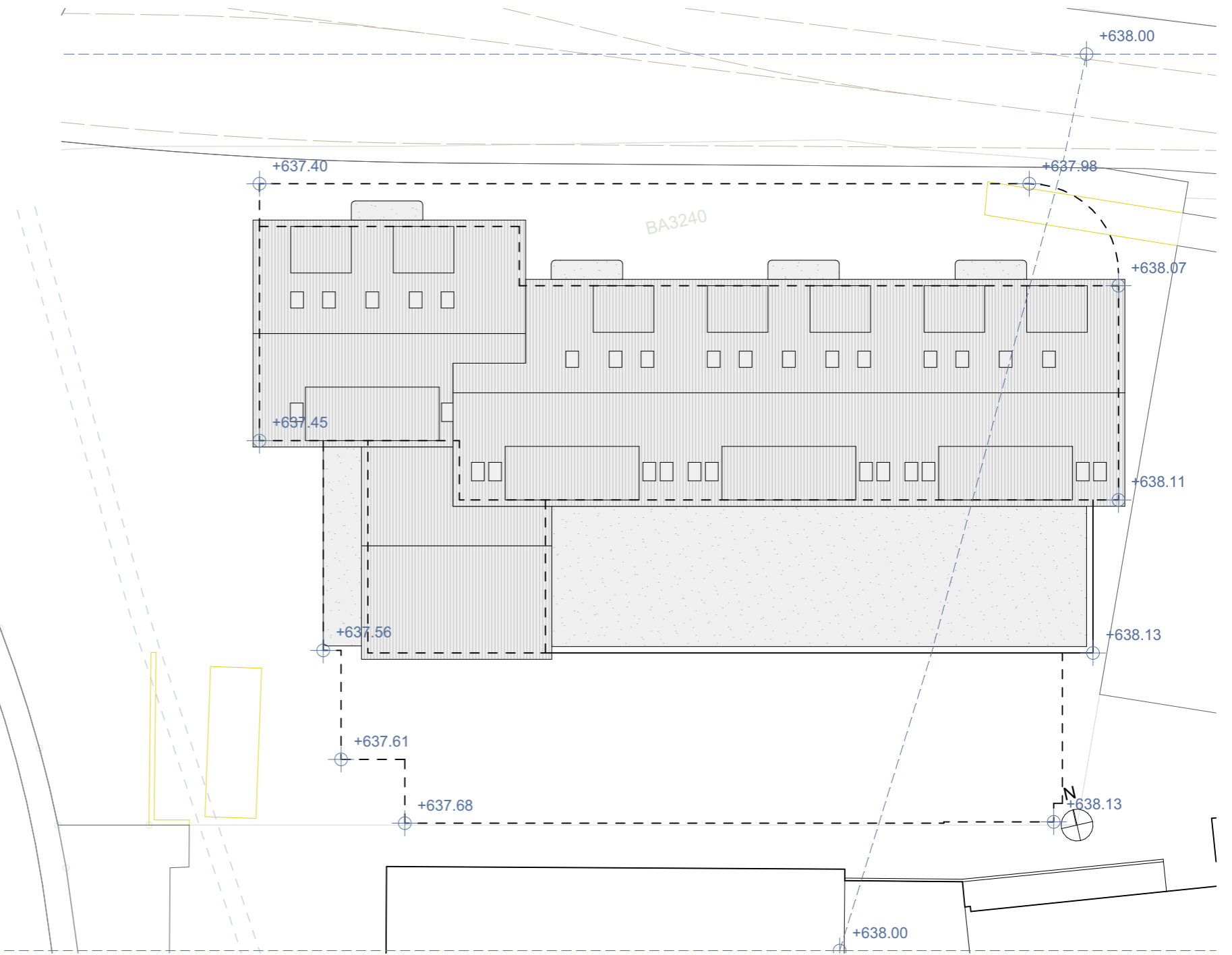
Isohypsen des mutmasslichen mittleren Grundwasserspiegels gem. Messungen der Firma Jäckli Geologie AG (17.11.2021)
